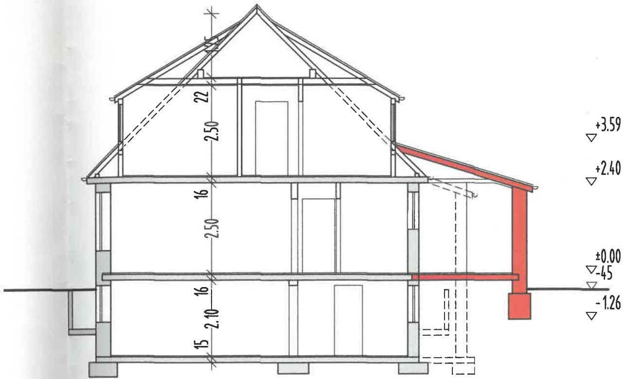
SCHNITT A - B
